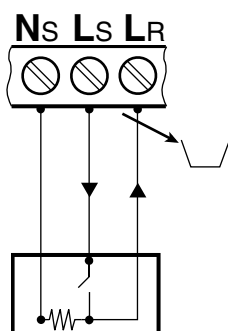
obr. 15 Připojení pokojového termostatu 230 V (odstraňte propojku mezi LS a LR)
