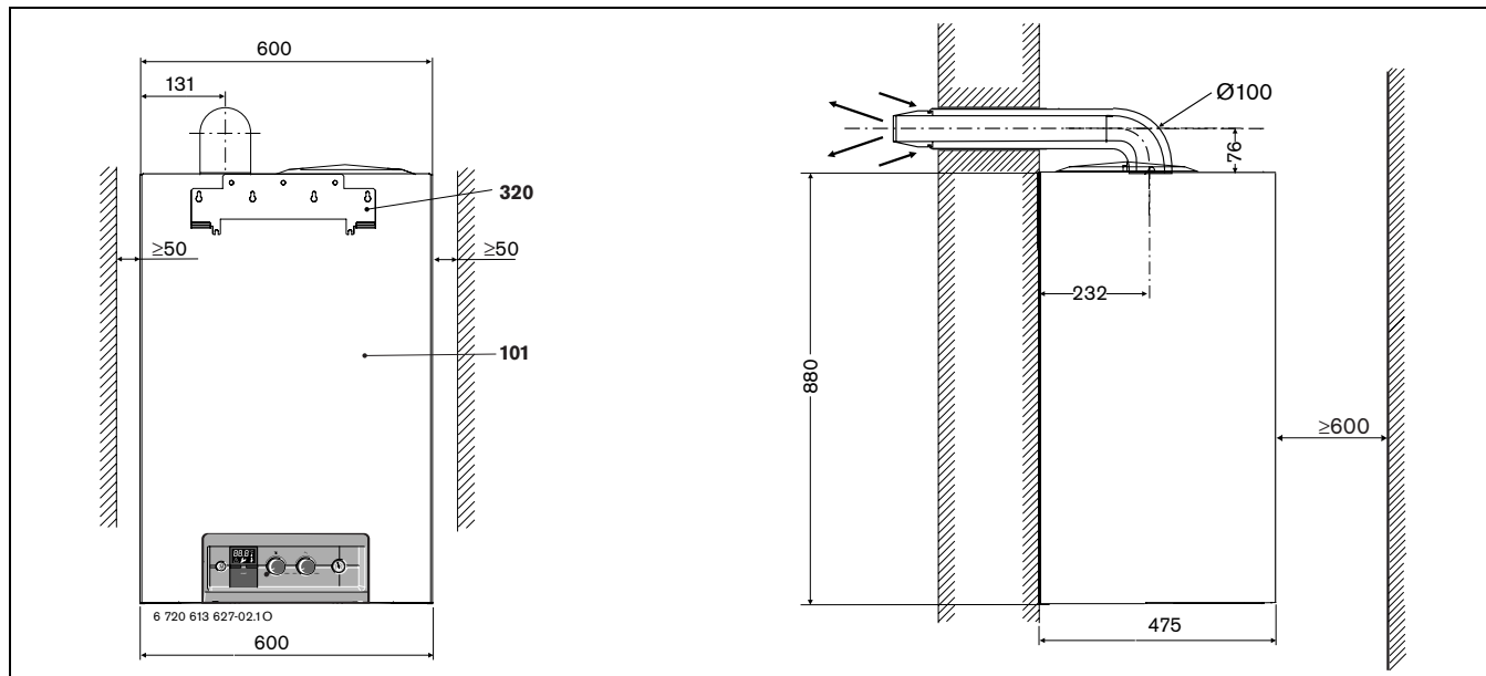
Obr. 2 DAGAS BT (odvod spalín dozadu)
