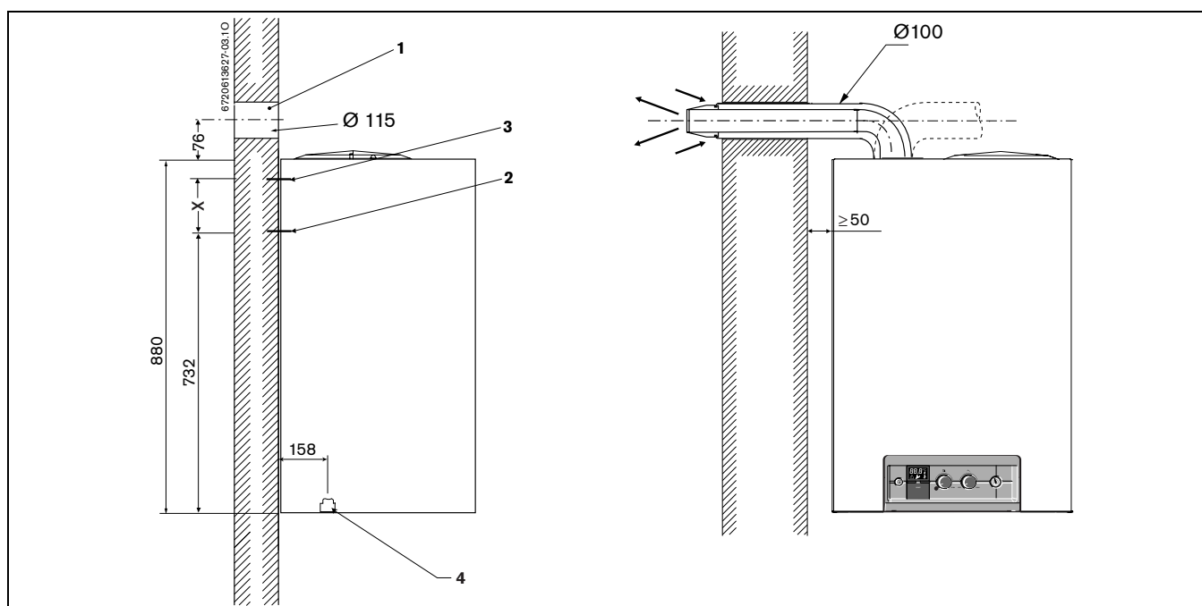
Obr. 3 DAGAS BT (odvod spalín po straně)
